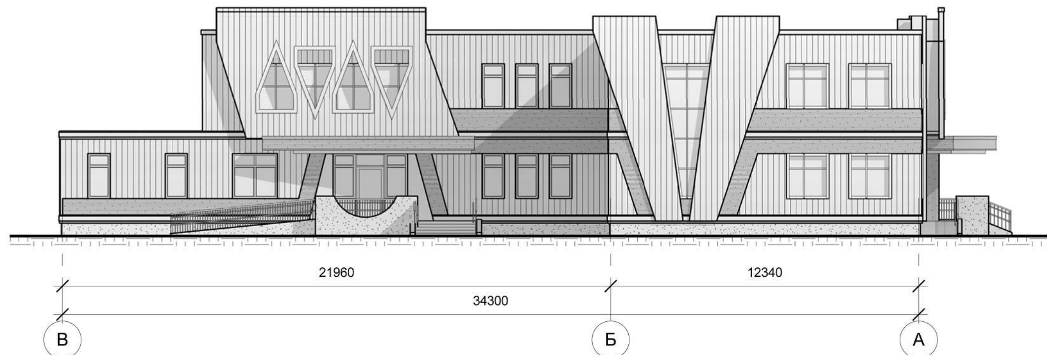
Фасад в осях В-А
